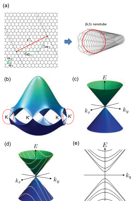
図 4. (a) グラフェンと CNT の構造の関係の模式図. 例としてカイラル指数 (n, m) = (6, 5) で指定される CNT の場合を図示した. \mathbf{C}_h (赤矢印) はカイラルベクトル. (b) グラフェンの分散関係の立体図. 点線で囲んだ部分は、K または K' バレーに対応する. (c) K または K' バレー近傍の線形な分散関係 (ディラックコーン) の模式図. (d) グラフェンの分散関係上に描いた半導体型 CNT の分散関係 (黄色線). CNT 軸の方向を k_y 方向、円周方向を k_x 方向に取った. (e) 典型的な半導体 CNT の分散関係.
