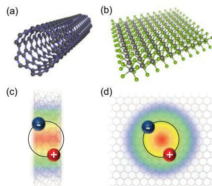
図 1. (a)単層カーボンナノチューブ, (b) 単層遷移金属ダイカルコゲナイドの模式図. (c), (d) それぞれの物質中の励起子の模式図.
