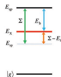
図 6. E_b , \Sigma , E_x , E_{qp} , E_{sp} の関係.
