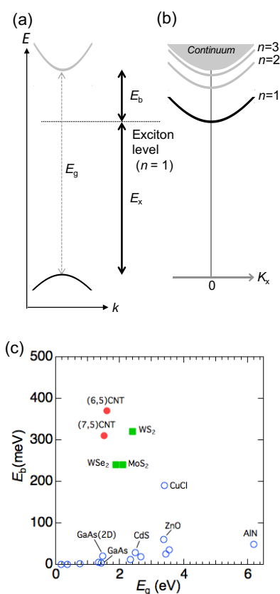
図 2. (a)直接半導体におけるバンドギャップ E_g と、励起子結合エネルギー E_b 、励起子エネルギー E_x の一般的な関係。 (b)励起子バンドの模式図。 (c)様々な直接ギャップ半導体の E_g と E_b の関係。
